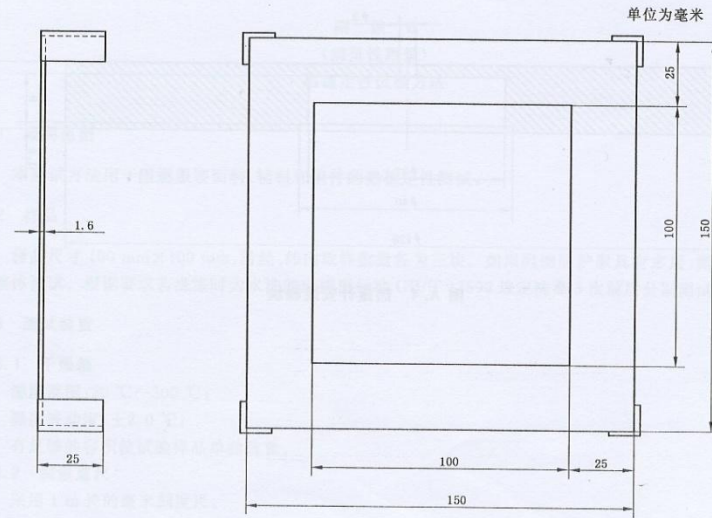
图 A.2 样品安装板的规格
