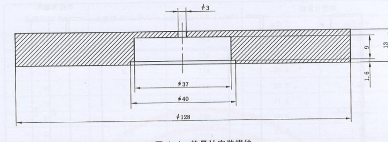
图 A.4 热量计安装模块
