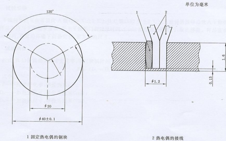
图 A.3 热量计
